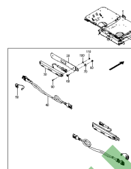
ETB-001087, Zestaw oświetleniowy do rozsiawacza przedniego
