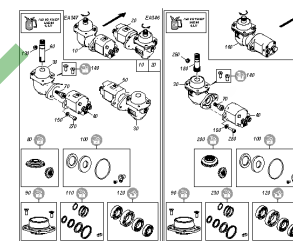
ETB-001128, Zewnętrzna skrzynia biegów Hydro - EA346/EA347
