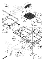
ETB-001064, ZA Super / Ultra / Special - rama i zbiornik
