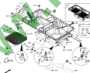
ETB-0000001463, ZA Super Profis (1)
