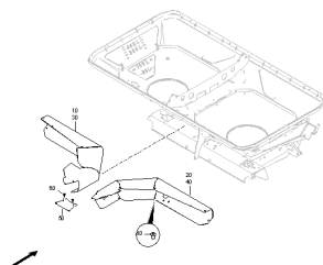
ETB-001065, Osłona przeciwbryzgowa jednoczęściowa
