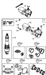
ETB-0000011484, Skrzynia biegów zewnętrzna hydrauliczna (przesuwna) w prawo
