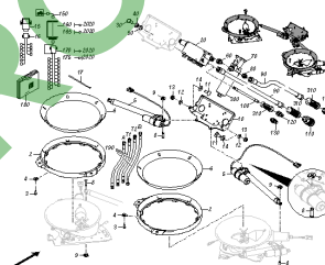
ETB-001114, Streuwiek TS Hydro El. Jednostka-PKT (3)
