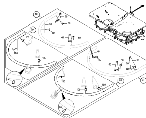
ETB-001160, Podwójne rury oporowe Argus
