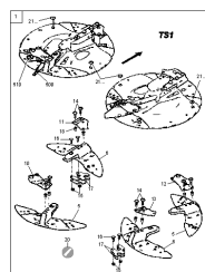
ETB-001105, Zestaw łopatek rozśiewających TS1, elementy montażowe
