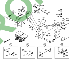
ETB-0000001501, Rama nakładkowa Ultra Quickhitsch
