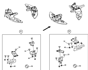
ETB-0000005149, Zestaw normalnych łopatek rozsiewających TS10
