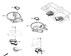
ETB-001097, Zestaw podłogowy TS (1) do 12-2023
