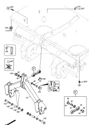
ETB-001063, ZA-Ultra bez techniki ważenia
