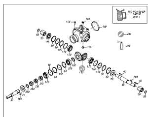
ETB-0000011557, Centrala skrzyni biegów 22,6 KW
