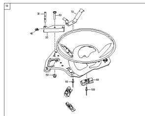
ETB-0000012966, Montaż podłogowy po lewej stronie
