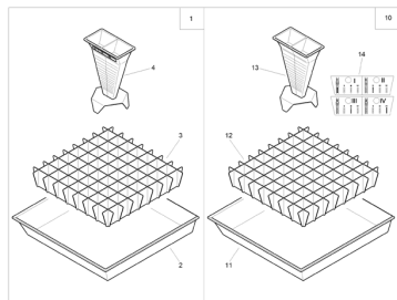
ETB-001181, Ruchome stanowisko pomiarowe
