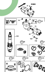
ETB-0000010269, Zewnętrzna hydrauliczna skrzynia biegów EA344/EA345
