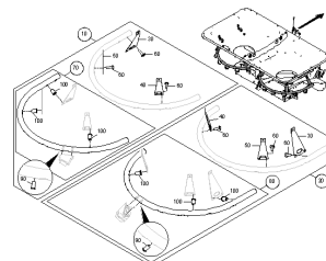
ETB-001160, Podwójne rury oporowe Argus
