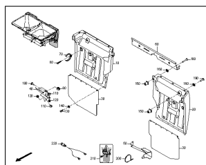
ETB-0000001164, Osłona przeciwbłotna S
