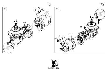
ETB-001132, Skrzynia biegów Hydro CFC
