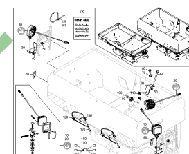
ETB-0000009399, Zestaw oświetlenia roboczego
