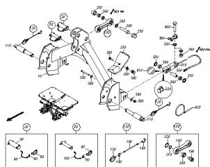
ETB-0000001501, Rama nakładkowa Ultra Quickhitsch
