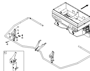
ETB-001189, Zestaw montażowy do ZA zawieszanego z przodu
