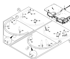
ETB-001160, Podwójne rury oporowe Argus
