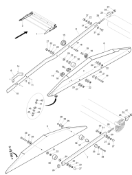
ETB-001172, Plandeka zwijana - szczyt do 12.2014
