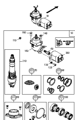
ETB-001129, Zewnętrzna hydrauliczna skrzynia biegów (przełączana)
