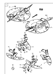
ETB-001111, Zestaw łopatek rozśiewających TS3, elementy
