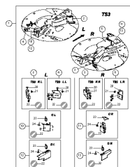
ETB-001113, Zestaw łopatek do rozsiewu granicznego TS3
