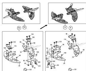
ETB-0000006992, Zestaw łyżek rozrzucających TS20
