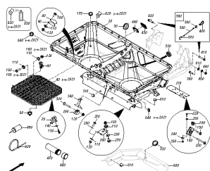
ETB-0000001624, ZA Super
