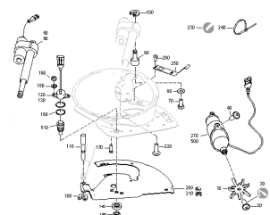
ETB-001094, Dno z otworami Tronic, jedn. el. PKT (2)
