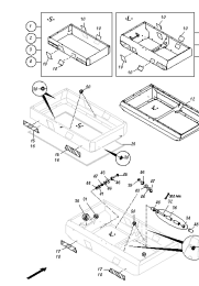
ETB-001073, Przystawka spawana S/L
