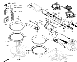
ETB-001100, Montaż podłogowy Hydro El. Wprowadzający PT (3)
