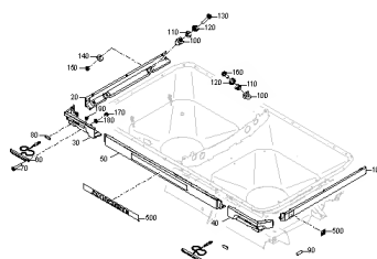
ETB-0000001212, Oświetlenie ledowe
