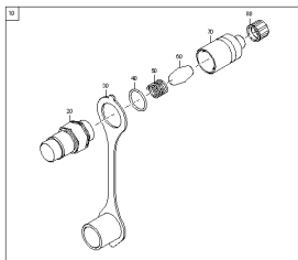
ETB-0000008845, Złącze SVK 12,5 z filtrem
