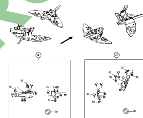
ETB-0000005156, Zestaw łopatek do rozsiewu granicznego TS20
