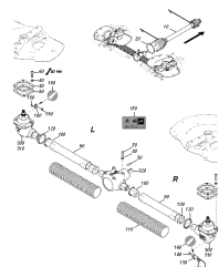
ETB-001122, TS napęd mechaniczny - wał napędowy / skrzynia biegów do 31.03.2025
