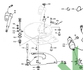
ETB-001091, Mechanizm rozsiewający TS Hydro, jedn. el. PKT (2)
