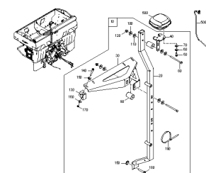
ETB-0000006208, Uchwyt na odbiornik GPS
