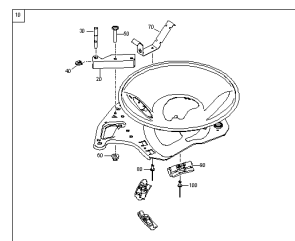
ETB-0000012966, Montaż podłogowy po lewej stronie
