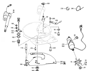
ETB-001119, Dno z otworami Tronic, jedn. el. PKT (2)
