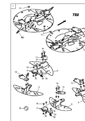
ETB-001108, Zestaw łopatek rozśiewających TS2, elementy montażowe
