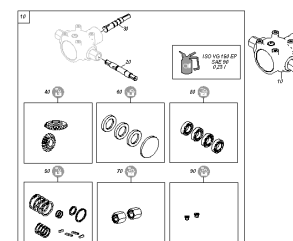
ETB-001125, Przekładnia środkowa 24 kW - EA341
