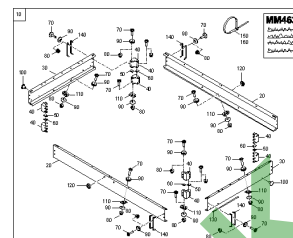
ETB-0000011631, Przedłużenie osprzętu S 600
