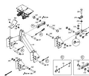
ETB-0000005074, Rama nakładkowa i komponenty zamienne System waż. Ultra Profis
