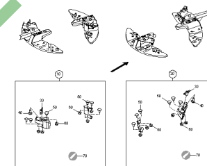
ETB-0000005150, Zestaw łopatek do rozsiewu granicznego TS10
