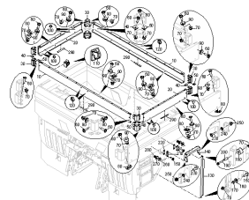
ETB-0000010593, Przedłużenie osprzętu L 800
