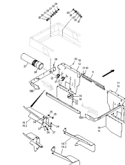
ETB-001085, Belka oświetlenia / osłona przeciwbłotna
