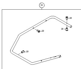
ETB-0000009339, Listwa ochronna rury S lewa
