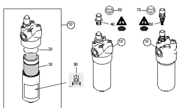
ETB-006791, Filtr hydrauliczny ciśnieniowy
