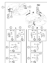
ETB-001107, Zestaw łopatek do rozsiewu granicznego TS1
