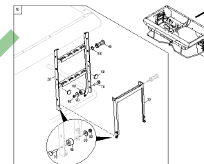
ETB-001080, Drabina od 02/2018
