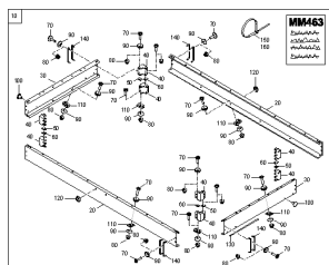
ETB-0000011629, Przedłużenie osprzętu L 800
