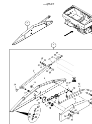
ETB-001177, Plandeka zwijana S i L hydrauliczna - szczyt lewy do roku prod. 2013
