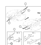
ETB-001108, Zestaw łopatek rozśiewających TS2, elementy montażowe
