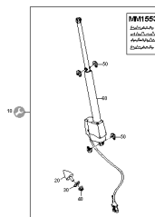
ETB-0000010693, Zestaw naprawczy Windcontrol
