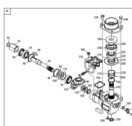
ETB-0000010456, Skrzynia biegów mech. Kontrola przepływu
