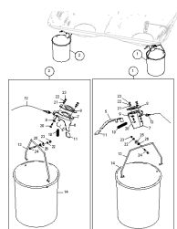
ETB-001180, Urządzenie do ustawiania odpowiedniej dawki rozsiewu
