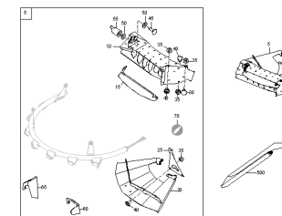
ETB-0000000908, Ekran rozsiewu granicznego
