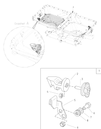
ETB-001069, Zestaw modernizacyjny do blokady ekranu
