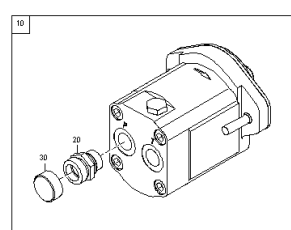
ETB-0000009675, Silnik hydrauliczny 17.3 prawy
