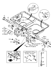
ETB-001067, Elementy ramowe
