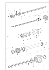
ETB-001124, Wałek przekąźnikowy EJ630
