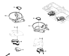
ETB-001101, Montaż podłogowy Hydro El. Absolutorium PKT (1) od 01.2020 r.
