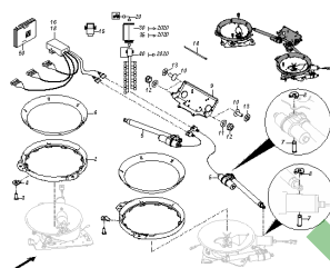
ETB-001092, Montaż podłogowy Tronic El. Jednostka-PKT (3)
