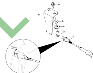
ETB-0000012320, Czujnik do sygnalizacji położenia dyfuzora
