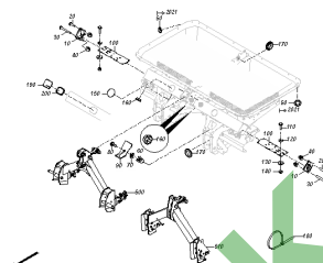
ETB-001071, ZA Ultra Profis (2)
