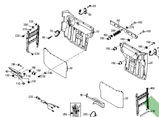
ETB-0000001169, Osłona przeciwbłotna i drabina L
