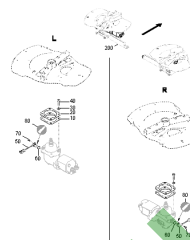
ETB-001123, Napęd TS hydrauliczny - Skrzynia biegów
