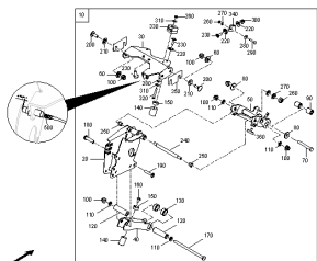
ETB-0000000840, Wspornik dyfuzora hydrauliczny (1)
