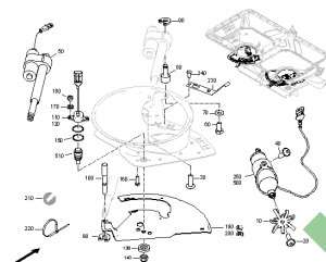
ETB-001116, Rozsiewacz TS Hydro El. Einheit-PKT (2) do 12.2019
