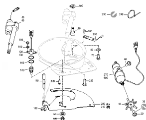
ETB-001102, Montaż podłogowy Hydro El. Absolutorium PKT (2) z dnia 01.2020 r.
