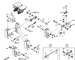
ETB-0000005074, Rama nakładkowa i komponenty zamienne System waż. Ultra Profis
