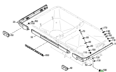
ETB-0000001177, Oświetlenie z żarówką do rocznika model. 2020 włącznie
