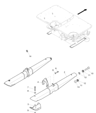
ETB-001175, Plandeka zwijana S i L hydrauliczna - szczyt lewy od 01.2015
