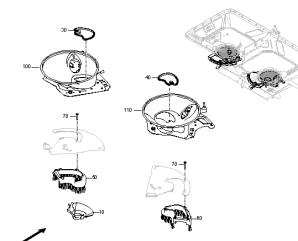
ETB-001118, Montaż podłogowy Tronic El. Absolutorium PKT (1) do dnia 12-2023 r.
