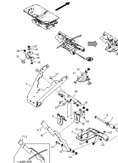
ETB-001183, Konsola ekranu rozsiewu ręczna
