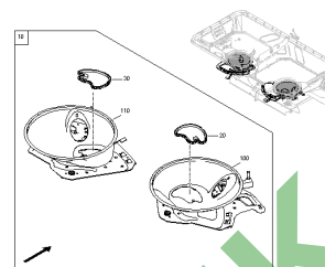
ETB-001103, Zestaw podłogowy TS MIDI (1) do 12-2023
