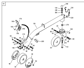
ETB-001424, Urządzenie toczone jednostronne
