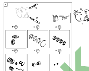
ETB-001125, Przekładnia środkowa 24 kW - EA341
