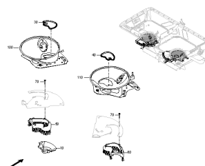
ETB-001090, Rozsiewacz TS Hydro El.Unit PKT (2)
