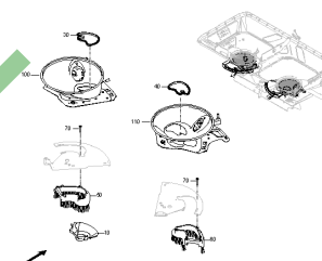
ETB-001093, Montaż podłogowy Tronic El. Jednostka-PKT (1) do 12-2023
