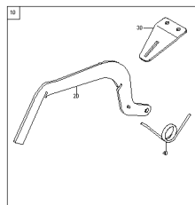
ETB-0000009517, Zestaw modernizacyjny man. Wspornik dyfuzora
