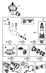
ETB-001127, Skrzynia biegów zewnętrzna mechaniczna (przełączana)
