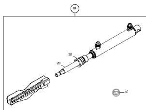
ETB-0000009127, Siłownik hydrauliczny
