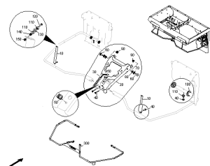
ETB-0000010173, Listwa ochronna rury L
