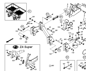
ETB-0000001291, ZA Super Profis (2)
