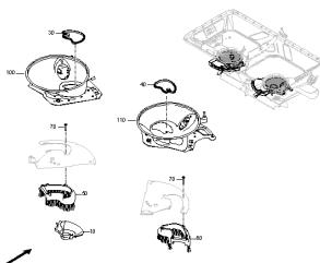
ETB-001115, Streuwiek TS Hydro El. Dział PTS (1) do 12.2019 do 12-2019
