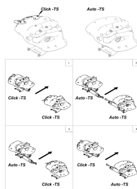
ETB-001121, Przegląd napędu TS hydraulicznego
