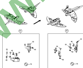
ETB-0000005162, Zestaw łopatek
