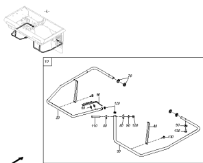
ETB-0000001155, Listwa ochronna rury L
