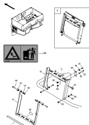
ETB-001083, Drabina S
