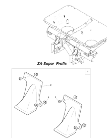
ETB-001068, Zestaw naprawczy do osłony ZA Super Profis
