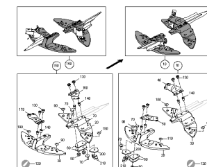
ETB-0000006993, Zestaw łyżek rozrzucających TS30
