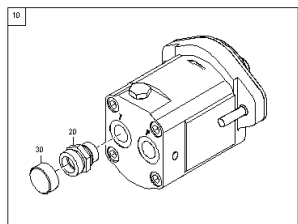
ETB-0000009673, Silnik hydrauliczny 17.3 Lewy
