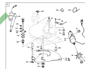
ETB-001104, Zestaw z dnem z otworami TS MIDI (2)
