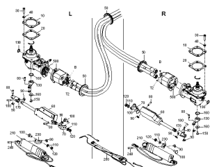
ETB-0000006111, Napęd Hydro Flow Control
