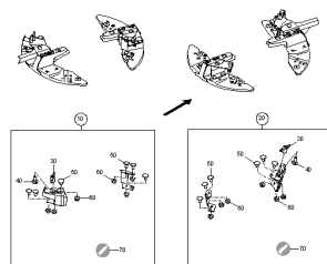
ETB-0000005150, Zestaw łopatek do rozsiewu granicznego TS10
