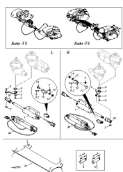
ETB-001135, Napęd TS - siłownik elektryczny
