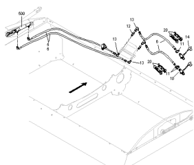
ETB-001175, Plandeka zwijana S i L hydrauliczna - szczyt lewy od 01.2015
