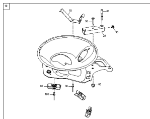
ETB-0000012967, Prawy montaż podłogi
