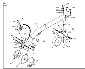
ETB-001424, Urządzenie toczne jednostronne
