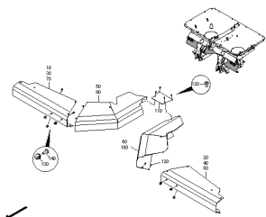
ETB-001066, Osłona przeciwbryzgowa dwuczęściowa
