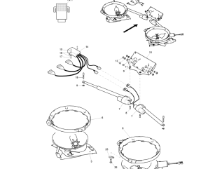
ETB-001096, Mechanizm rozsiewający ZA-TS elektryczny
