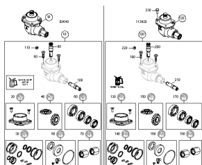
ETB-001126, Skrzynia biegów na zewnątrz 8 KW / 12 kW
