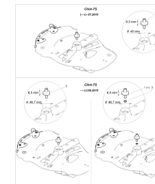
ETB-001139, Śruba zabezpieczająca do Click-TS
