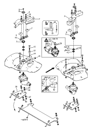
ETB-001136, Talerz główny - łopatki kierujące / osłona blaszana do przekładni zewnętrznej
