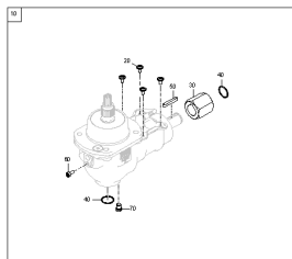
ETB-000000363, Przekładnia mechaniczna CFC
