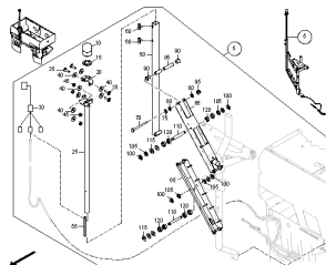
ETB-001078, Zestaw do konwersji Windcontrol
