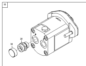
ETB-0000009675, Silnik hydrauliczny 17.3 prawy
