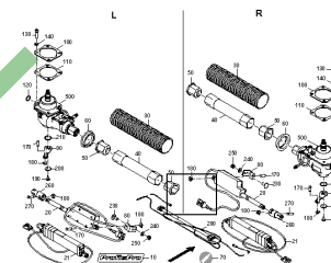
ETB-0000006109, Sterowanie przepływem napędu
