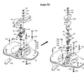
ETB-001137, Talerz główny (Auto- TS)
