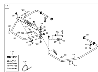
ETB-0000009338, Zestaw doposażeniowy w listwę ochronną rury S
