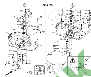
ETB-001138, Talerz główny (Click- TS) -- sterowanie ręczne
