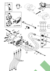
ETB-001141, Sterowanie ZA-TS Hydro
