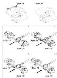
ETB-001120, Przegląd napędu TS mechanicznego
