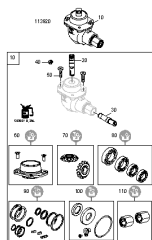
ETB-0000010910, Skrzynia biegów zewnętrzna 12 kW 113920
