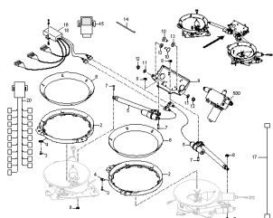
ETB-001089, Rozsiewacz TS Hydro El.Unit PKT (1)
