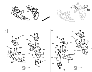
ETB-0000005147, Zestaw łopatek rozsiewających TS10, elementy montażowe
