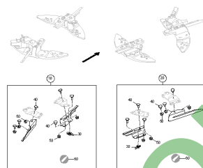
ETB-0000005153, Zestaw normalnych łopatek rozsiewających TS20
