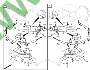
ETB-0000009517, Zestaw modernizacyjny man. Wspornik dyfuzora
