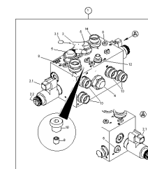
ETB-001142, Blok sterujący GD925
