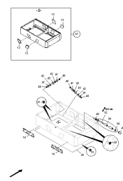
ETB-001072, Nadstawka S 2600 spawana
