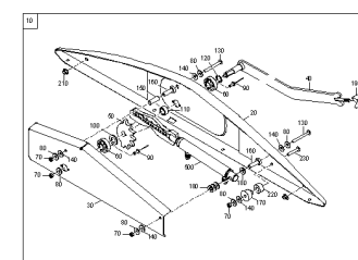
ETB-001178, Plandeka zwijana S i L hydrauliczna - szczyt lewy od roku prod. 2014
